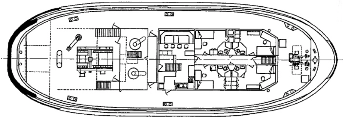
VUE SOUS PONT PRINCIPAL
