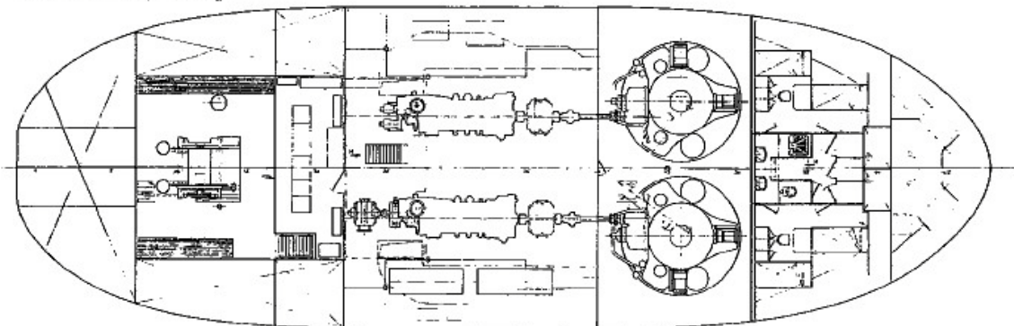
VUE SOUS PONT PRINCIPAL
